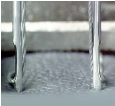
DRALLVERSCHUB
